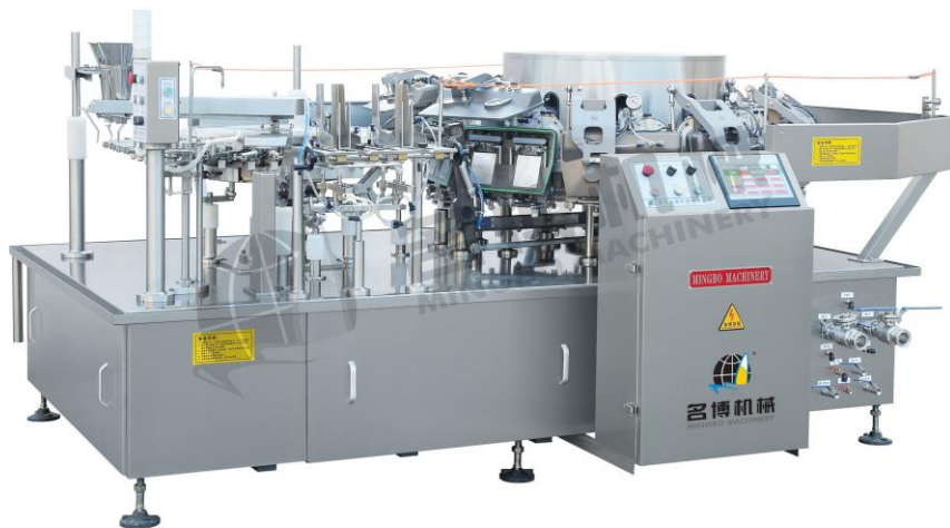
（雙給袋式自動真空包裝機）
