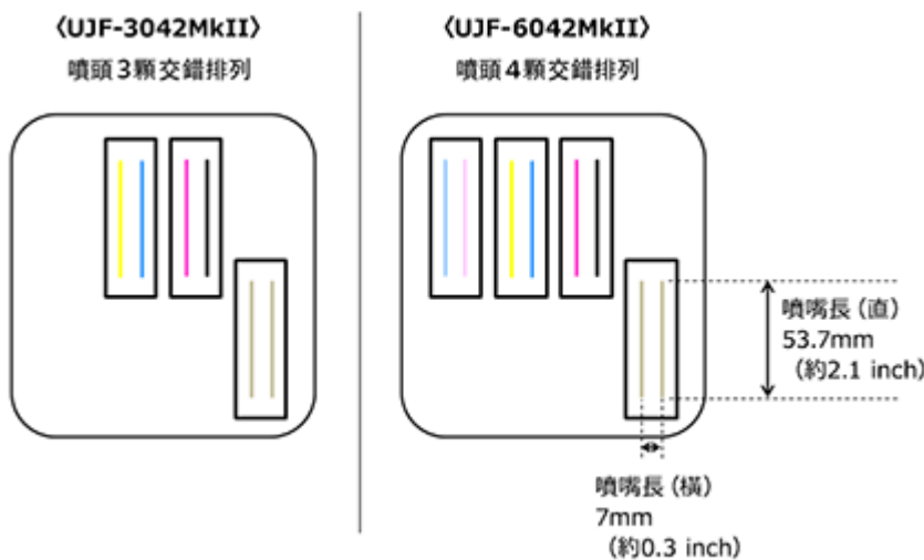
图 1 : 喷头配置示意图
